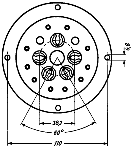
Fassung Lager-Nr. 30 229
