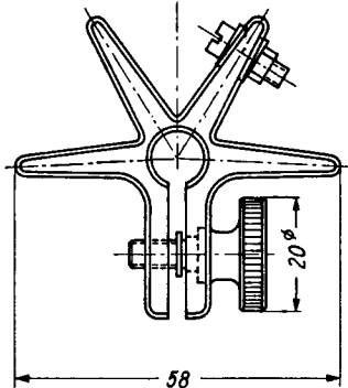
Anodenanschluß Lager-Nr. 30 393
