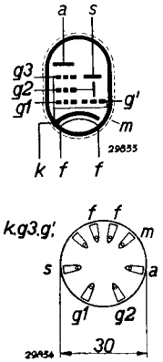
Abb. 2 Elektrodenanordnung und mit- und Sockelanschlüsse.
