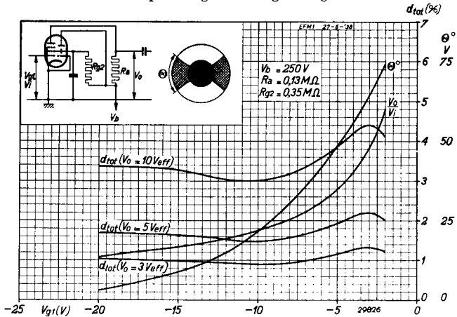
Abb. 5 Verzerrung als Funktion der Gittervorspannung mit der Ausgangswechselfspannung als Parameter bei R_{G_2} = 350.000 Ohm, R_a = 130.000 Ohm und V_b = 250 V und Schattenwinkel \Theta als Funktion der Gittervorspannung.
