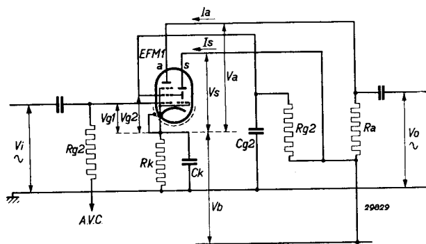
Abb. 6 Schaltung zur Erläuterung der in den Daten angegebenen Größen.
