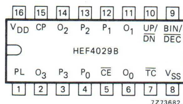
Fig. 2 Pinning diagram.
