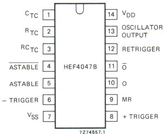
Fig. 2 Pinning diagram.
