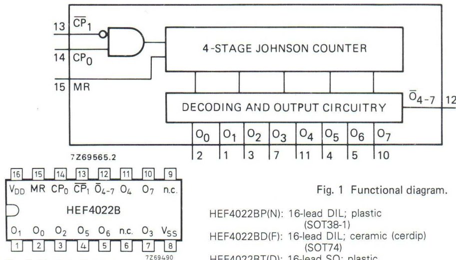
Fig. 2 Pinning diagram.
