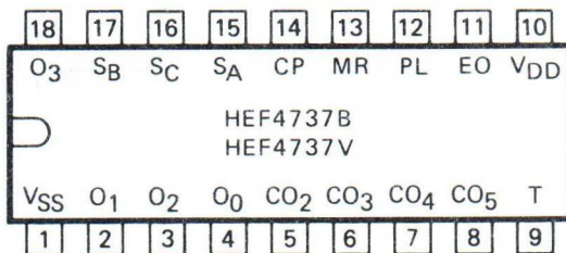
Fig. 1 Pinning diagram.
