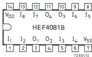
Fig.2 Pinning diagram.
