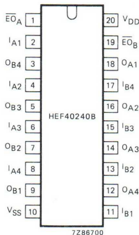
Fig. 2 Pinning diagram.
