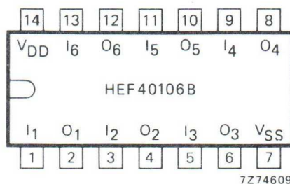
Fig. 2 Pinning diagram.
