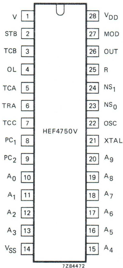
Fig. 1 Pinning diagram.
