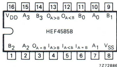
Fig. 2 Pinning diagram.
