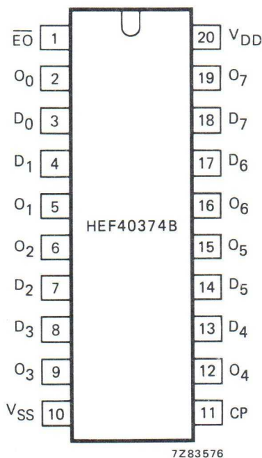
Fig. 2 Pinning diagram.
