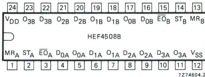
Fig. 2 Pinning diagram.
