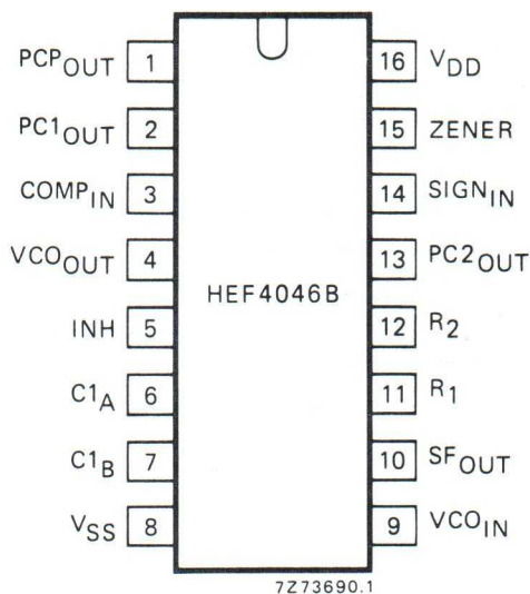
Fig. 2 Pinning diagram.
