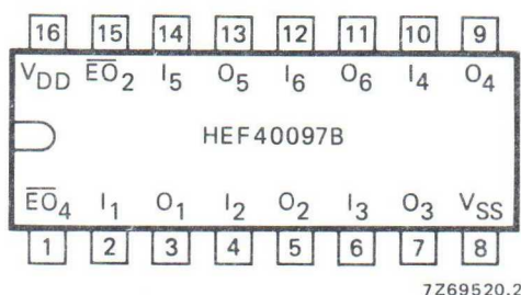
Fig. 2 Pinning diagram.
