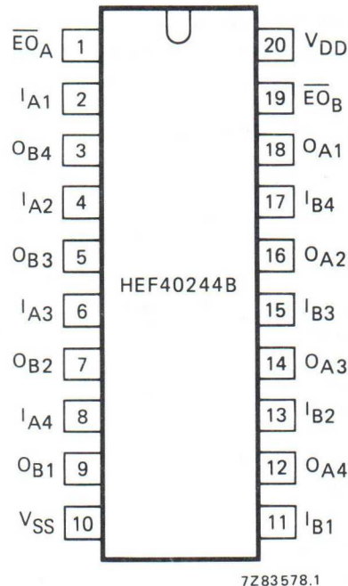
Fig. 2 Pinning diagram.
