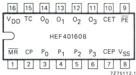
Fig. 3 Pinning diagram.
