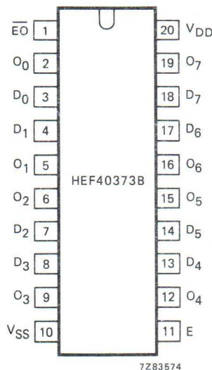
Fig. 2 Pinning diagram.
