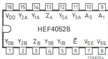
Fig. 2 Pinning diagram.
