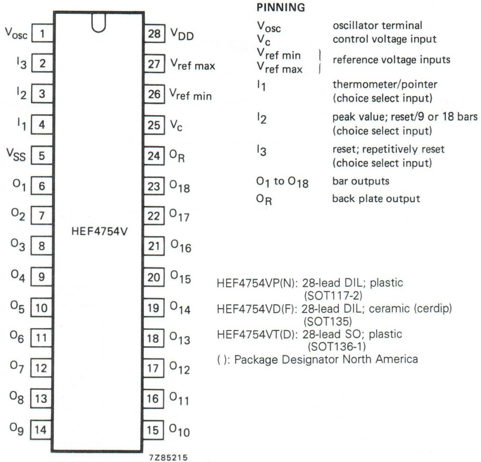
Fig. 2 Pinning diagram.
