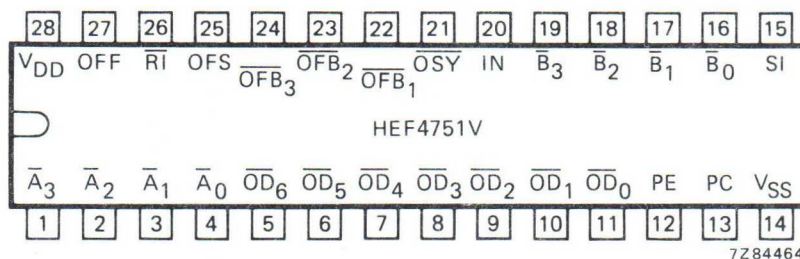
Fig. 1 Pinning diagram.
