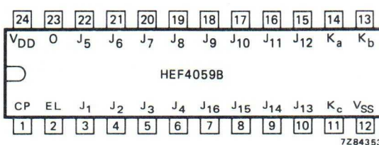
Fig. 2 Pinning diagram.
