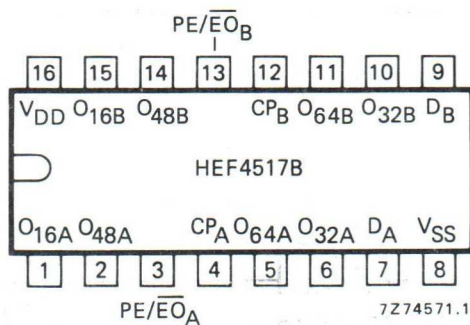
Fig. 2 Pinning diagram.
