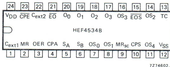
Fig. 1 Pinning diagram.
