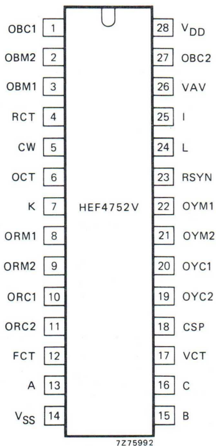
Fig. 1 Pinning diagram.
