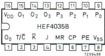
Fig. 3 Pinning diagram.
