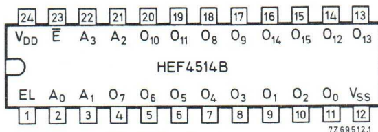
Fig. 2 Pinning diagram.
