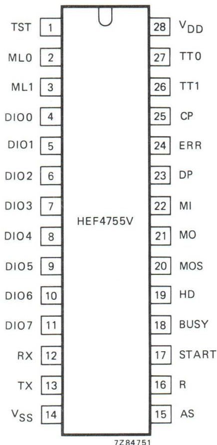
Fig. 1 Pinning diagram.
