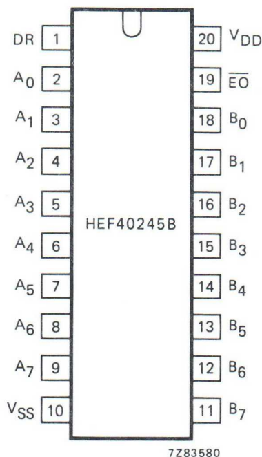
Fig. 1 Pinning diagram.
