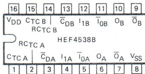
Fig. 2 Pinning diagram.
