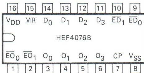
Fig. 2 Pinning diagram.
