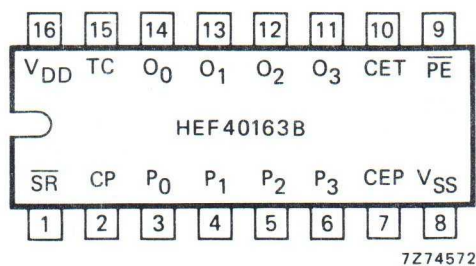
Fig. 3 Pinning diagram.
