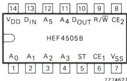
Fig. 1 Pinning diagram.
