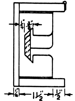
END ELEVATION
