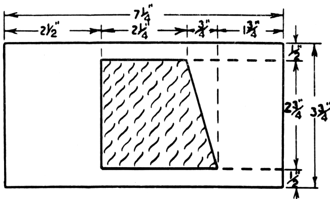
PLAN OF LID
