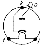
Sockelschaltenschema
